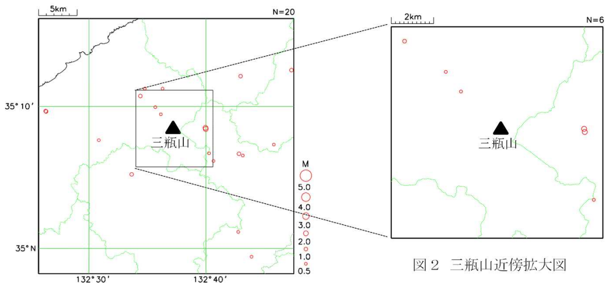
図1 三瓶山周辺の震央分布図 (2024年4月、M \geq 0.5、深さ0km \sim 30km)
