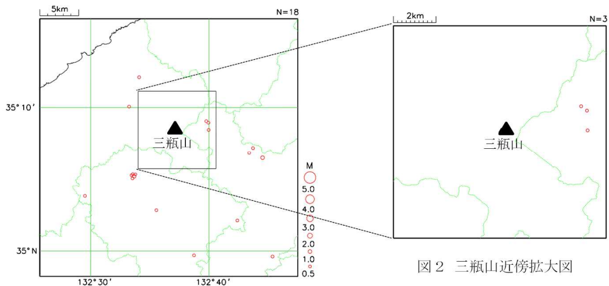
図1 三瓶山周辺の震央分布図 (2024年5月、M \geq 0.5、深さ0km \sim 30km)
