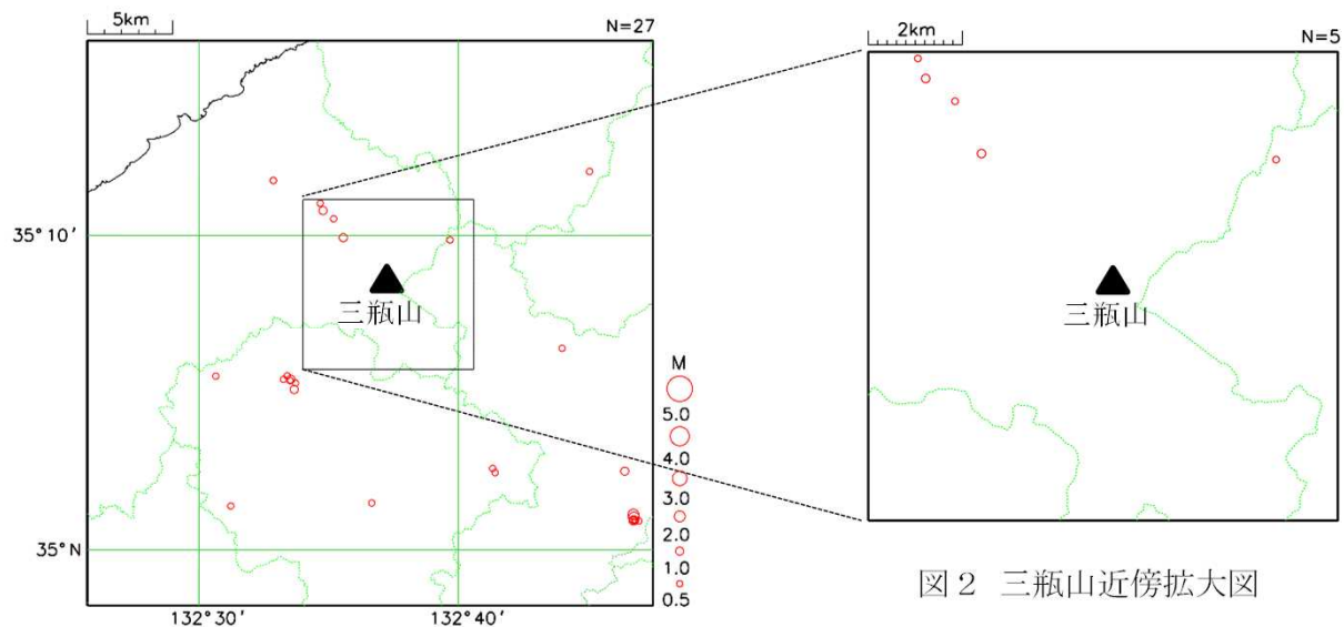
図1 三瓶山周辺の震央分布図 (2024年6月、M \geq 0.5、深さ0km \sim 30km)
