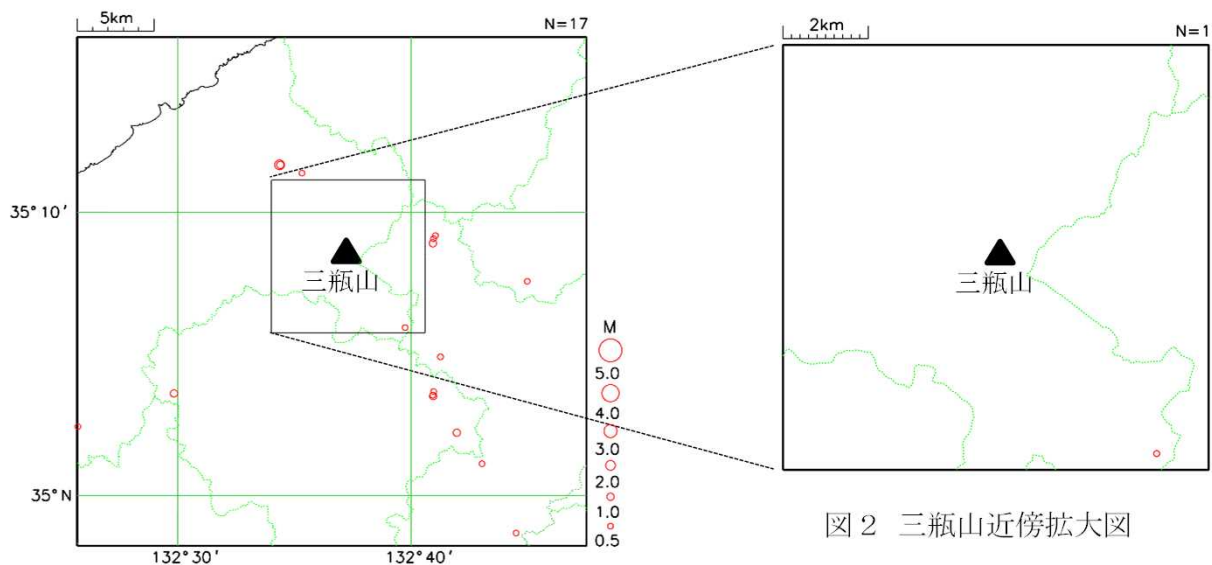
図 1 三瓶山周辺の震央分布図 (2024年10月、M \geq 0.5、深さ 0 km \sim 30km)
