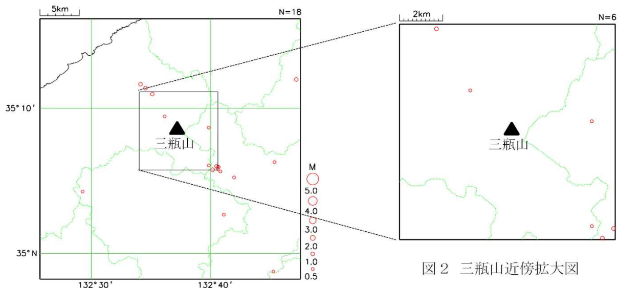
図 1 三瓶山周辺の震央分布図 (2024年11月、M \geq 0.5、深さ 0km \sim 30km)
