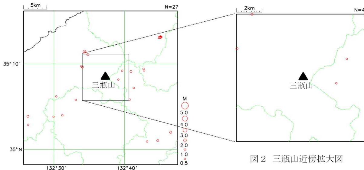
図 1 三瓶山周辺の震央分布図 (2024 年 12 月、 M \geq 0.5 、深さ 0 km ~ 30 km)
