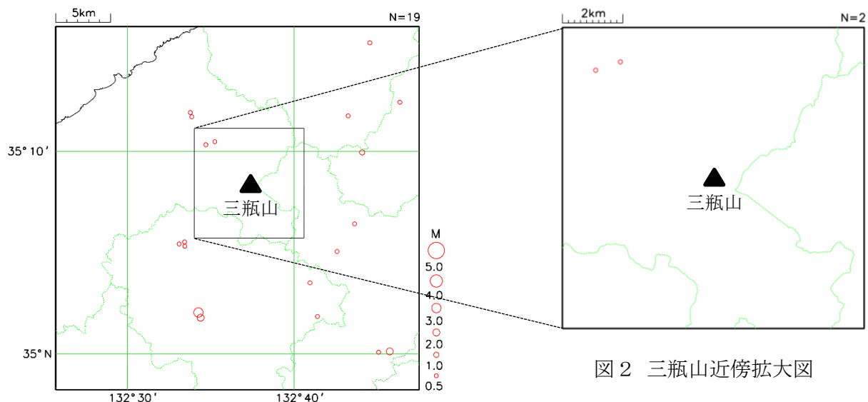
図1 三瓶山周辺の震央分布図 (2025年7月、M \geq 0.5、深さ0km \sim 30km)
