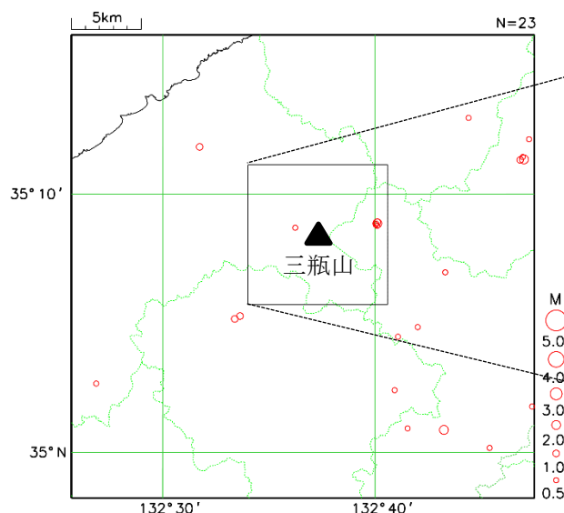
図 1 三瓶山周辺の震央分布図 (2025 年 8 月、M \geq 0.5、深さ 0 km \sim 30 km)
