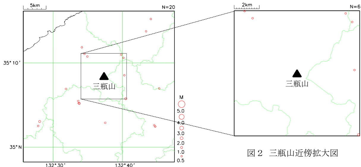
図 1 三瓶山周辺の震央分布図 (2025年10月、M \geq 0.5、深さ0km \sim 30km)
