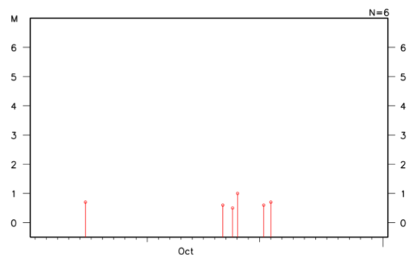
図 3 地震活動経過図（図 2 の領域内）
