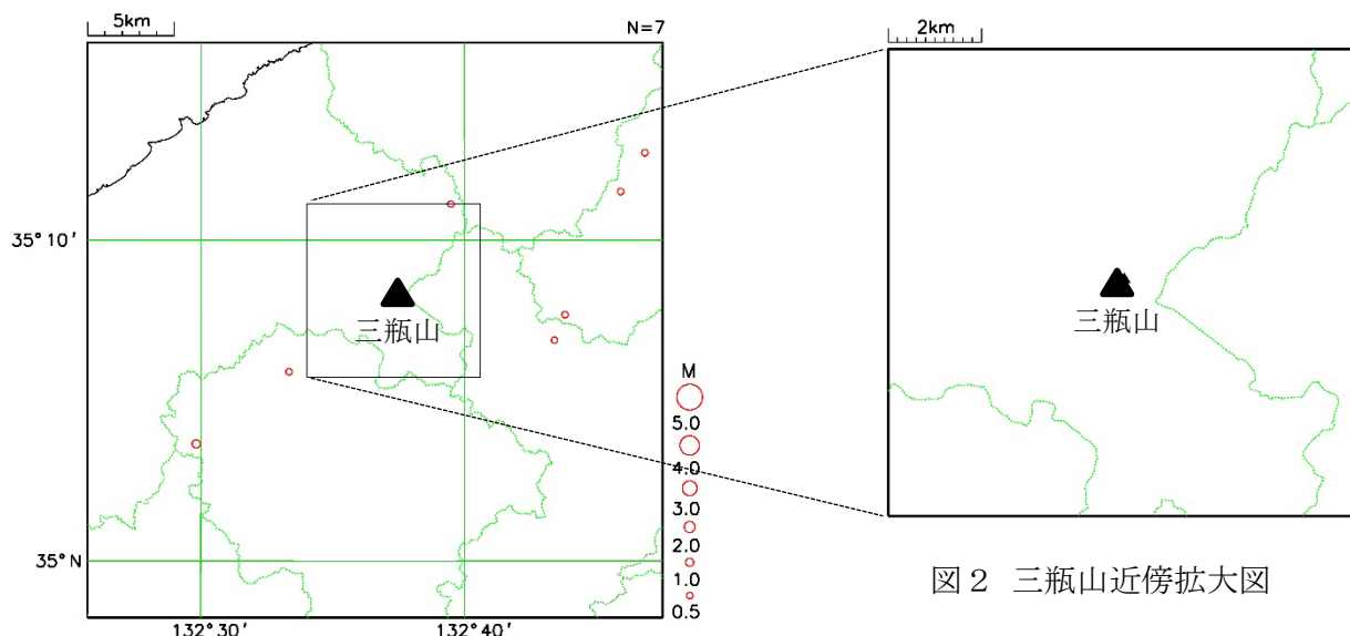
図1 三瓶山周辺の震央分布図 (2026年6月、M \geq 0.5、深さ0km \sim 30km)
