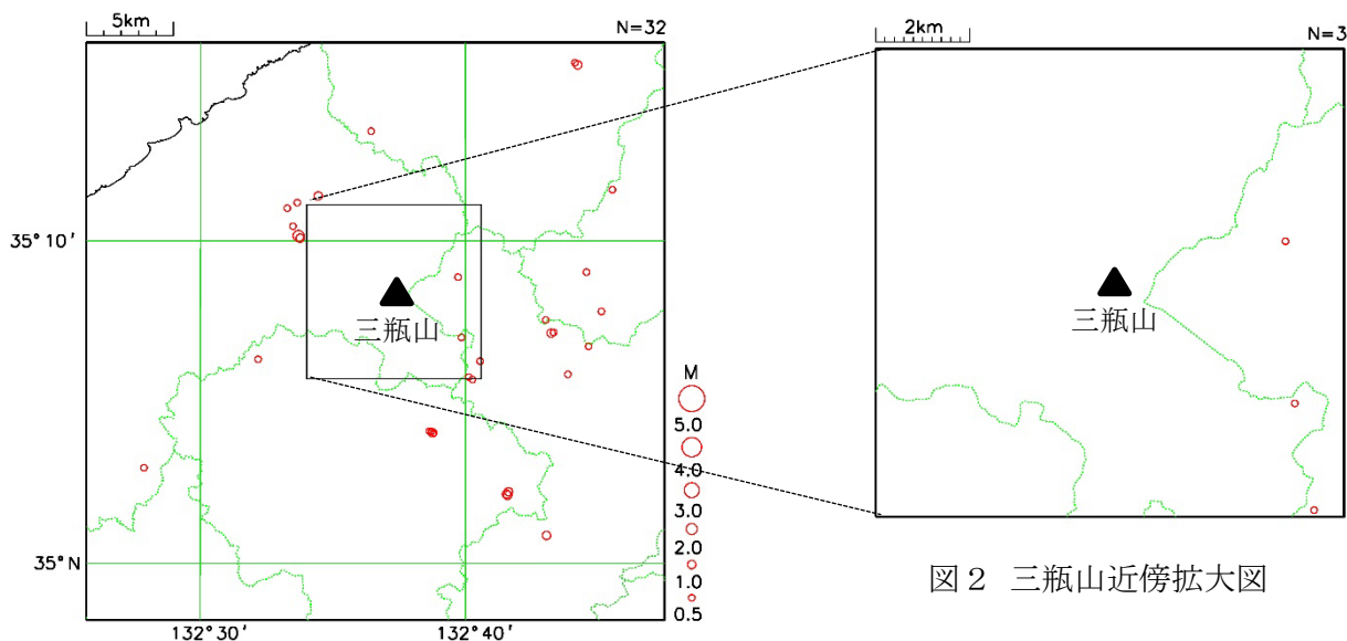
図1 三瓶山周辺の震央分布図 (2026年8月、M \geq 0.5、深さ0km \sim 30km)
