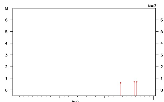
図3 地震活動経過図（図2の領域内）
