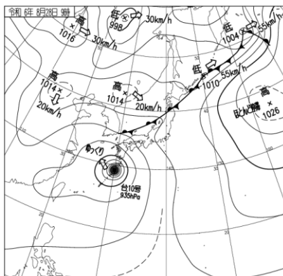
地上天気図
