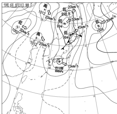
地上天気図
