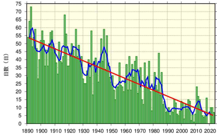
第 1 図 松山の年間冬日日数の経年変化(1890 年～2023 年)
