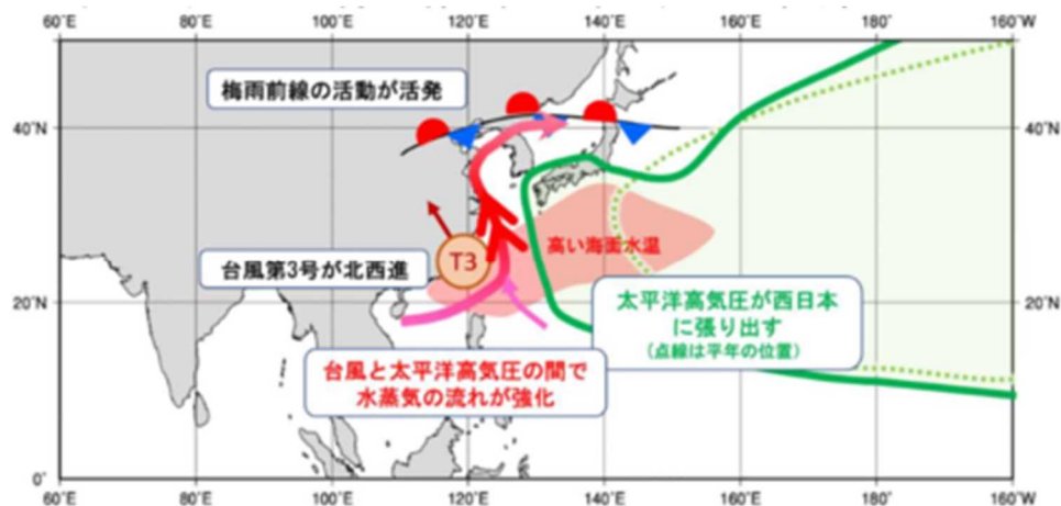
7月下旬に北日本に大雨をもたらした大規模な大気の流れに関する模式図
