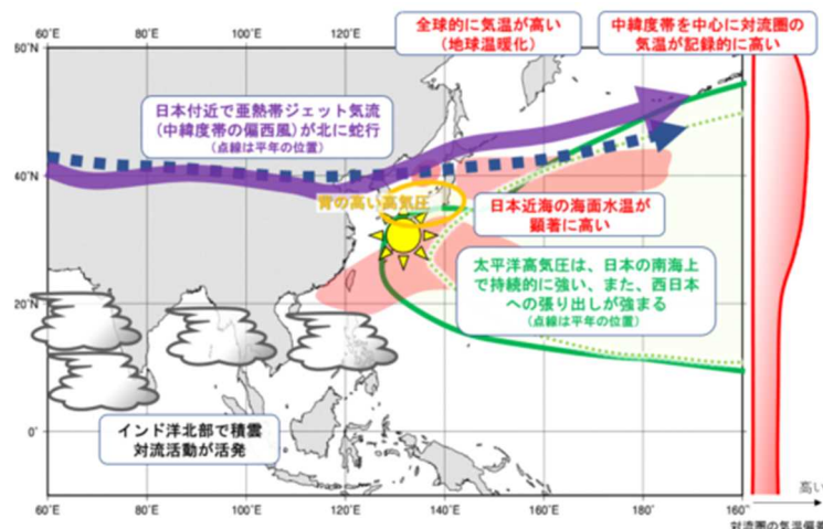
7月の顕著な高温をもたらした大規模な大気の流れに関する模式図
