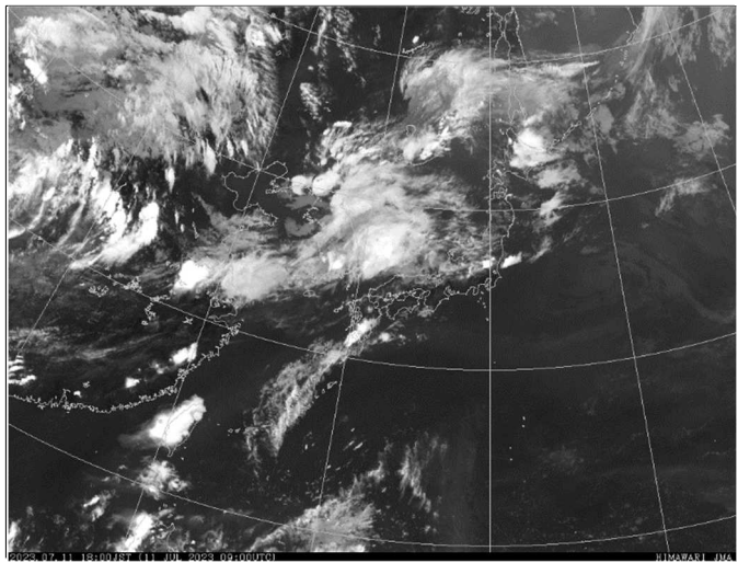
7月11日18時の地上天気図（左）と気象衛星赤外面像（右）
