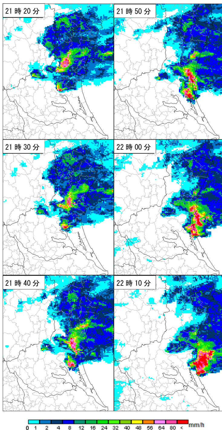
7月13日21時20分から10分毎のレーダー画像
