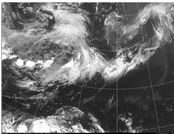
7月13日21時の地上天気図（左）と気象衛星赤外面像（右）
