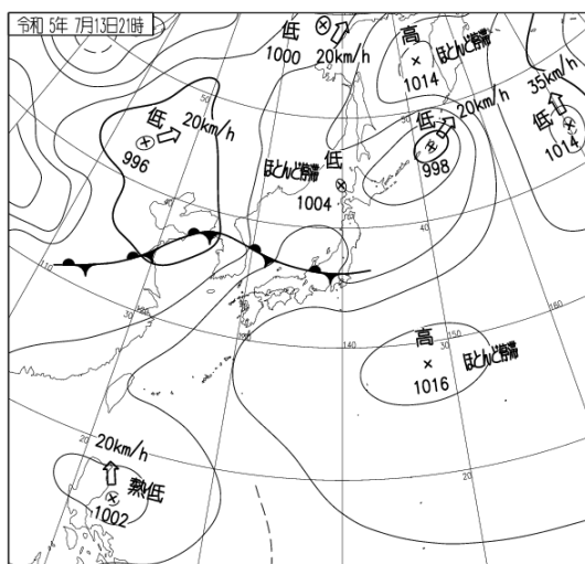
7月13日21時の地上天気図（左）と気象衛星赤外面像（右）
