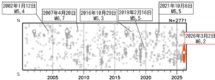
領域a内の時空間分布図 (南北投影)
