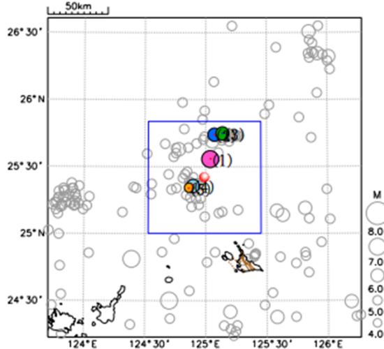
過去の主な地震
