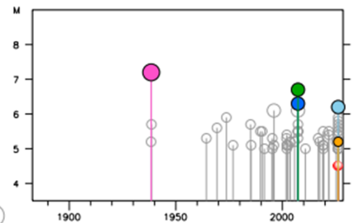
過去の主な地震
