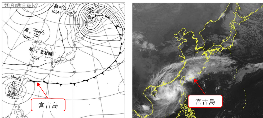
11月11日09時の地上天気図（左）と気象衛星赤外画像（右）
