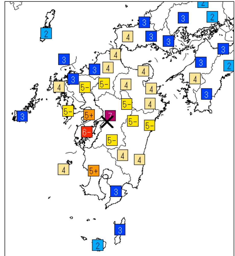
震度分布図（地域別）
