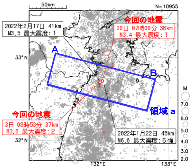
図2 震央分布図
