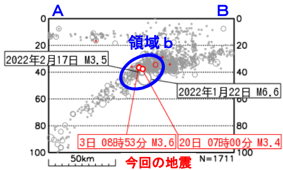
図3 図2領域a内の断面図 (A-B投影)
