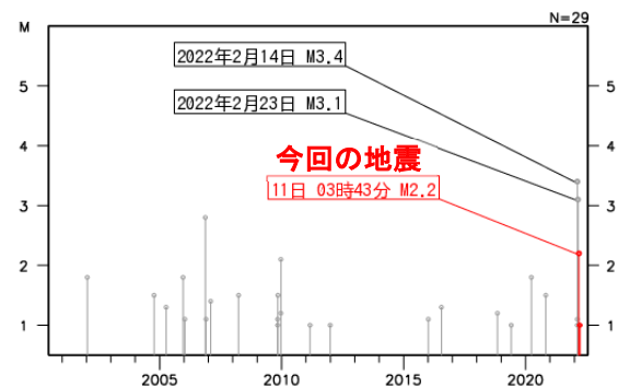
図 7 図 6 領域 a 内の地震活動経過図
