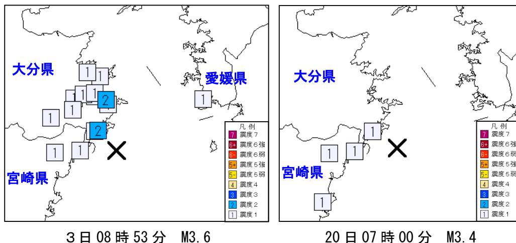
図 1 震度分布図（観測点別、×：震央）
