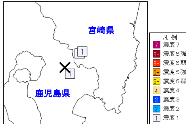
図 5 震度分布図（観測点別、×：震央）
