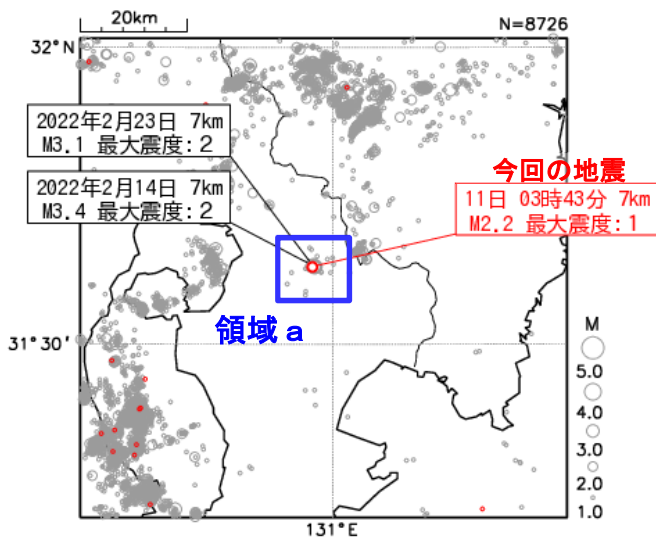
図 6 震央分布図 (2000 年 10 月 1 日～2022 年 3 月 31 日、 深さ 0～20 km、M ≥ 1.0) ※2022 年 3 月の地震を赤色で表示
