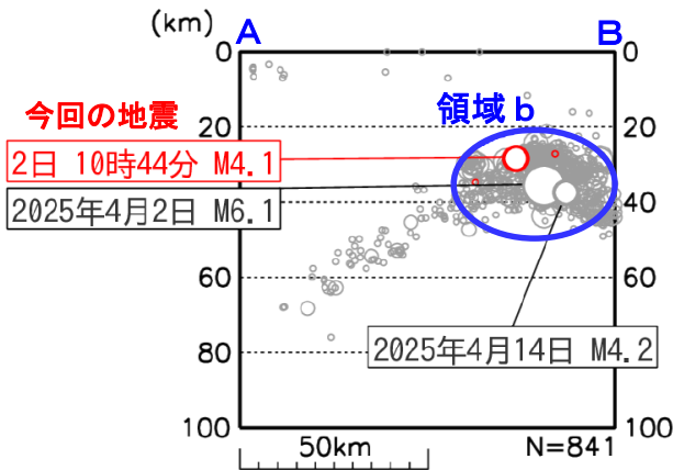
図 3 図 2 領域 a 内の断面図（A－B 投影）
