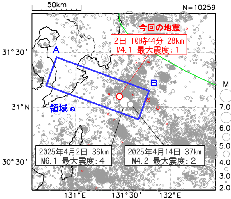
図 2 震央分布図
