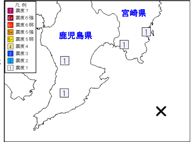
図 1 震度分布図（観測点別、×：震央）
