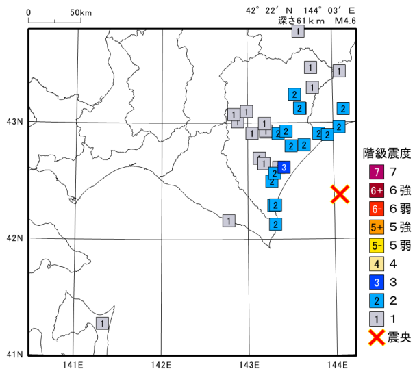
2022年 2月13日15時50分 十勝沖の地震の震度分布図
