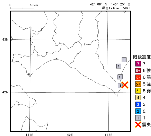
2022年 2月 11日 09時42分 十勝沖の地震の震度分布図
