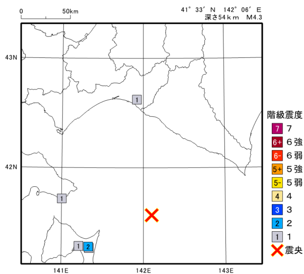
2022年 2月 6日 07時30分 青森県東方沖の地震の震度分布図
