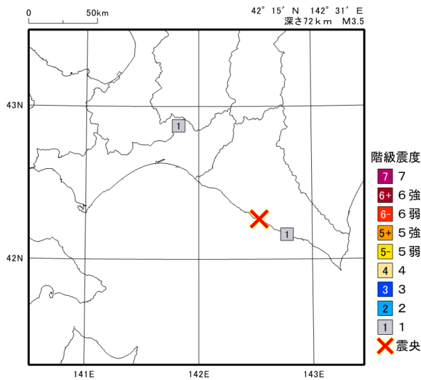
2022年 2月22日21時23分 浦河沖の地震の震度分布図
