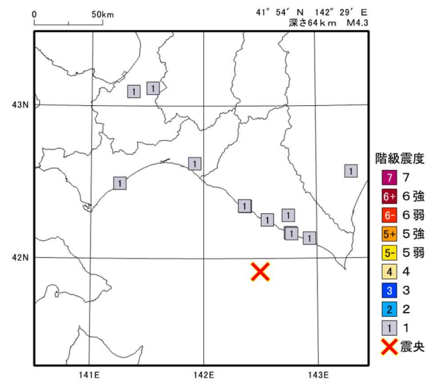
2024年 4月 15日01時06分 浦河沖の地震の震度分布図
