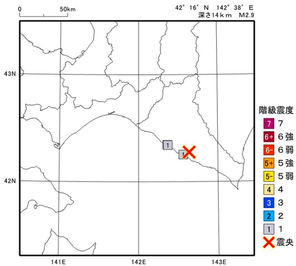
2024年 4月 29日12時54分 日高地方中部の地震の震度分布図
