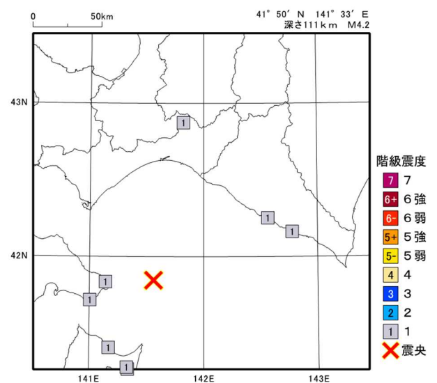
2024年 4月 4日 03時 09分 苫小牧沖の地震の震度分布図
