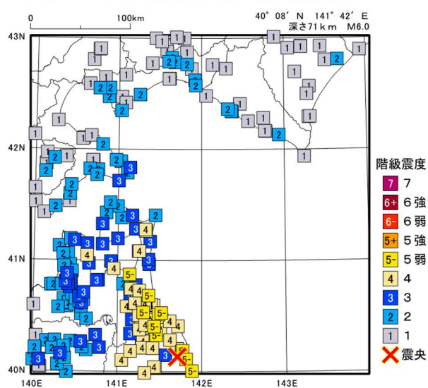
2024年 4月 2日 04時 24分 岩手県沿岸北部の地震の震度分布図
