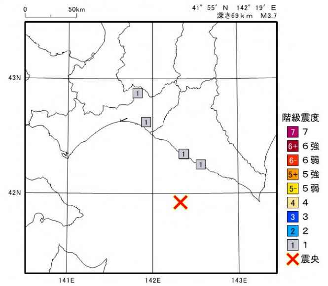
2024年 6月28日15時43分 浦河沖の地震の震度分布図
