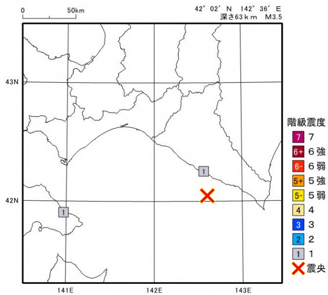
2024年 6月27日20時27分 浦河沖の地震の震度分布図
