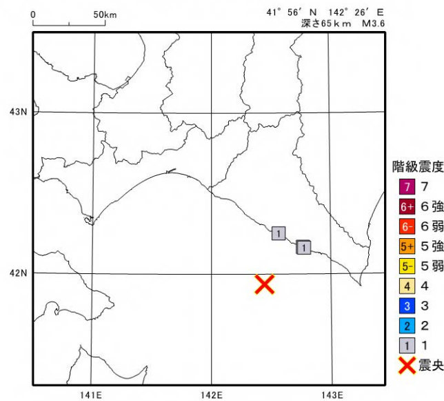
2024年 6月18日 01時31分 浦河沖の地震の震度分布図
