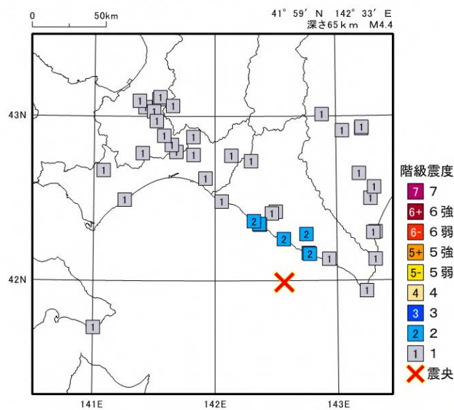
2024年 6月12日 14時35分 浦河沖の地震の震度分布図
