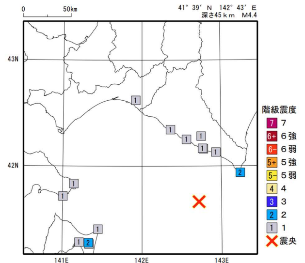
2024年 9月19日06時33分 浦河沖の地震の震度分布図
