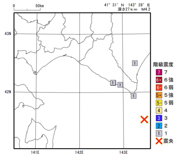
2024年 9月25日02時07分 十勝沖の地震の震度分布図
