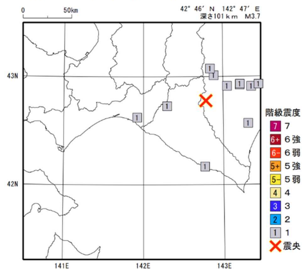
2024年9月14日13時46分 十勝地方中部の地震の震度分布図
