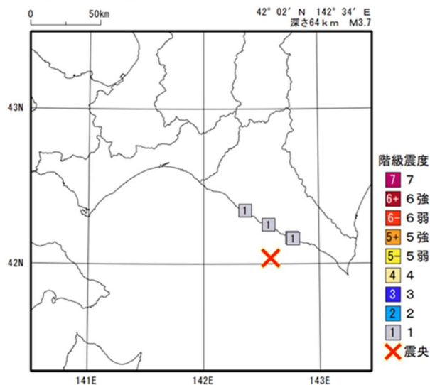
2024年 9月22日06時13分 浦河沖の地震の震度分布図
