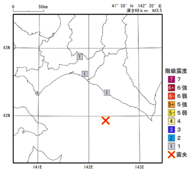
2024年9月12日13時08分 浦河沖の地震の震度分布図
