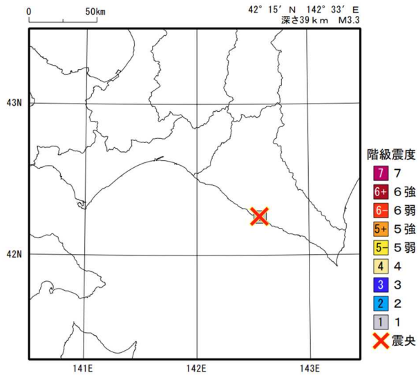
2024年 9月18日07時35分 日高地方中部の地震の震度分布図
