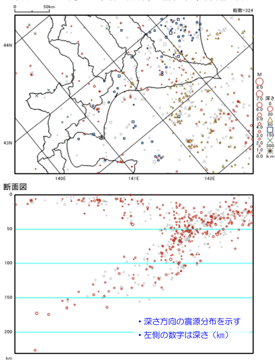
図２ 断面図の例
