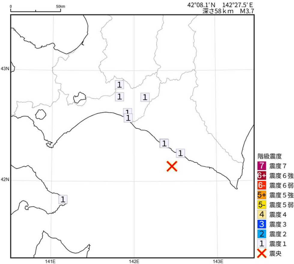
2025年9月4日 11時33分 浦河沖の地震の震度分布図
