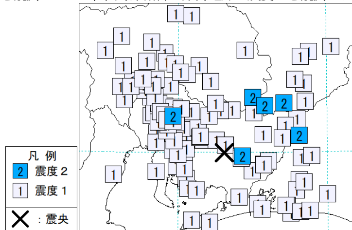
図4 11月30日 愛知県西部の地震の震度分布図(地点別)
