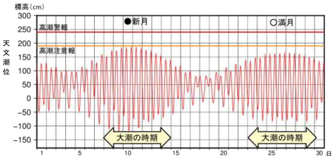
図3 長崎における2018年9月の天文潮位
