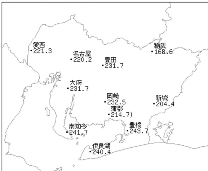
アメダス月別値 2019年8月 日照時間(h)
