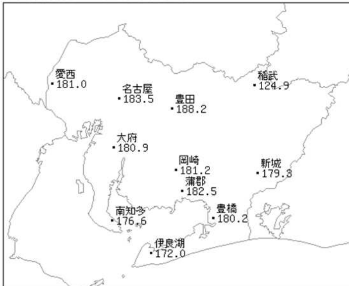
アメダス月別値 2018年11月 日照時間(h)
