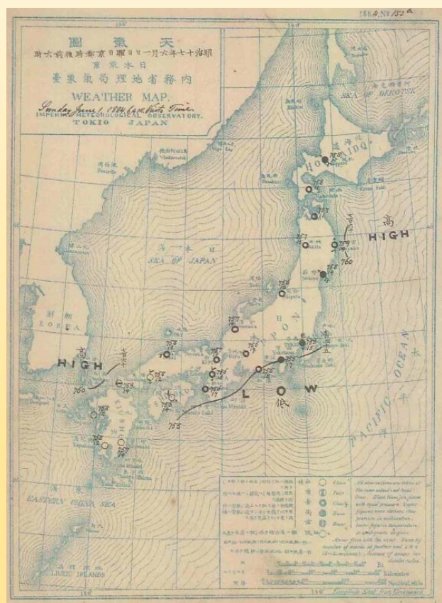
日本初の天気予報発表時の天気図 (明治17年6月1日6時)
