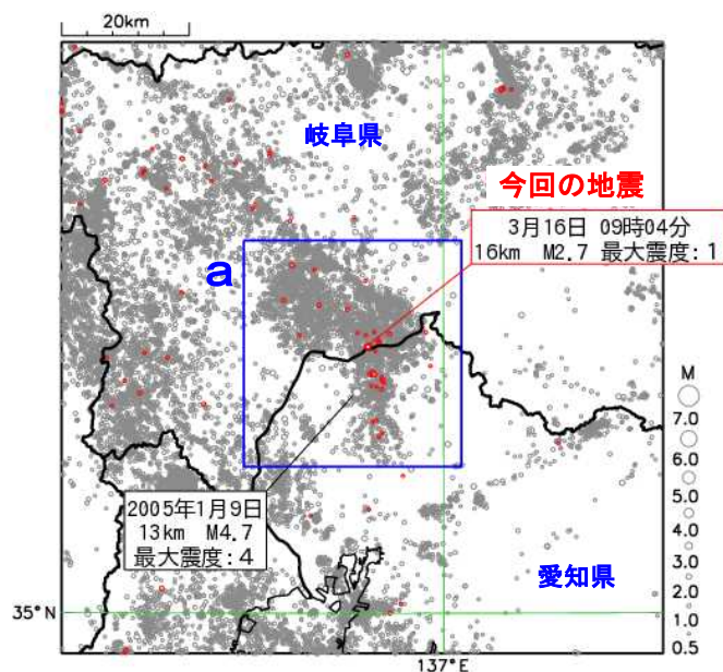
図2 震央分布図 （1997年10月1日～2021年3月31日 深さ0～20km M≥0.5） ※2021年3月の地震を赤で表示
