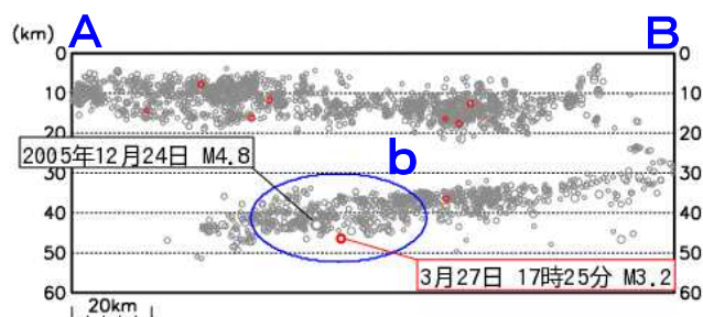
図3 領域a内の断面図（A－B投影）
