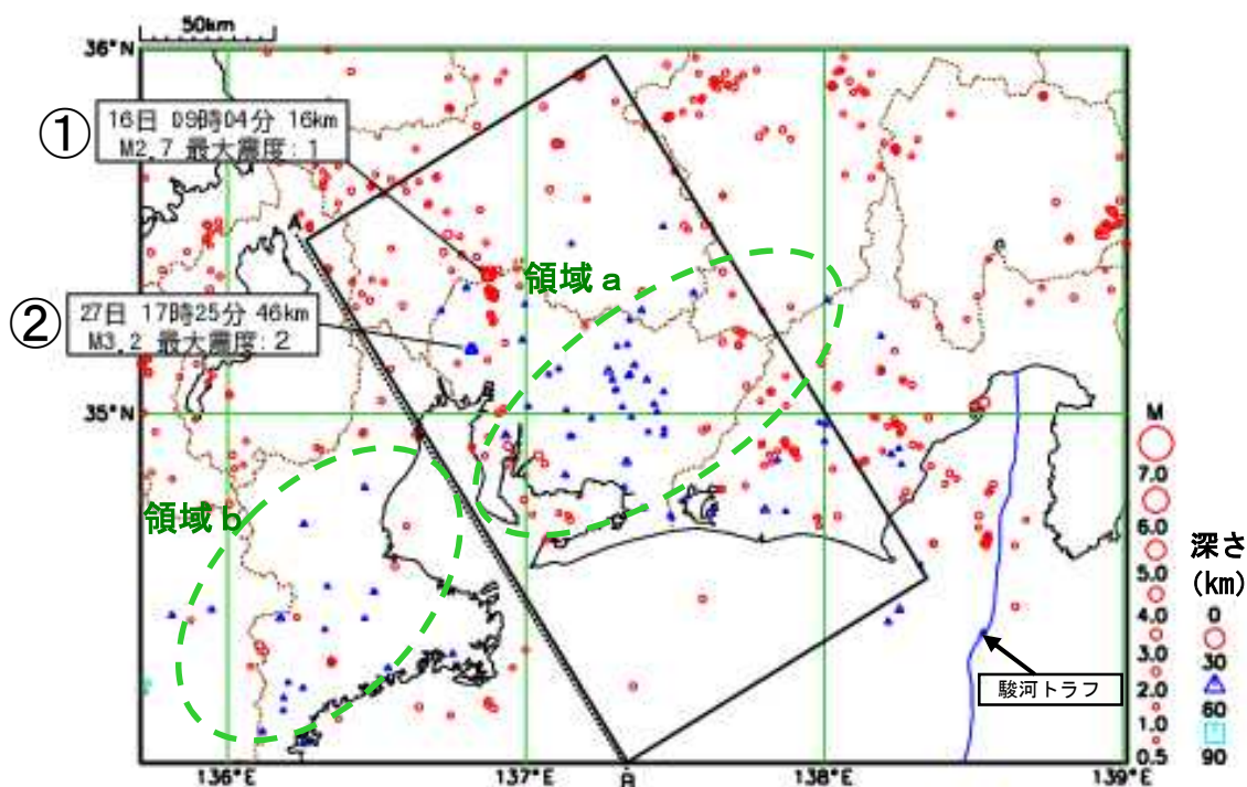
震央分布図（2021年3月1日～31日 深さ0～90km M \geq 0.5）
