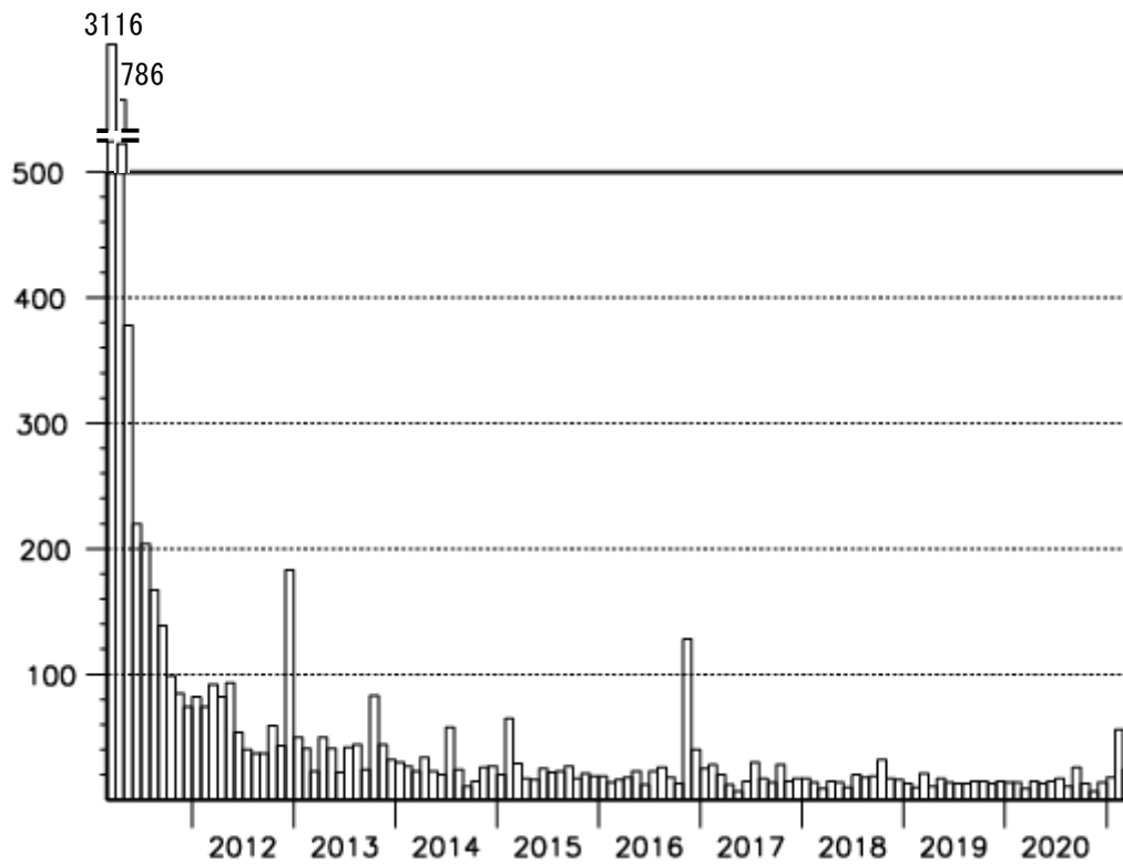
図4 領域a内の地震の月別回数 ( M \geq 4.0 )
