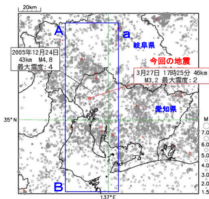
図2 震央分布図 （1997年10月1日～2021年3月31日 深さ0～60km M \geq 1.5） ※2021年3月の地震を赤で表示
