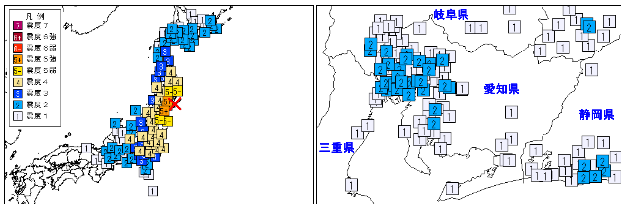
図1 3月20日18時09分 M6.9 震度分布図（×：震央、左図地域別の広域図、右図観測点別の詳細図）
