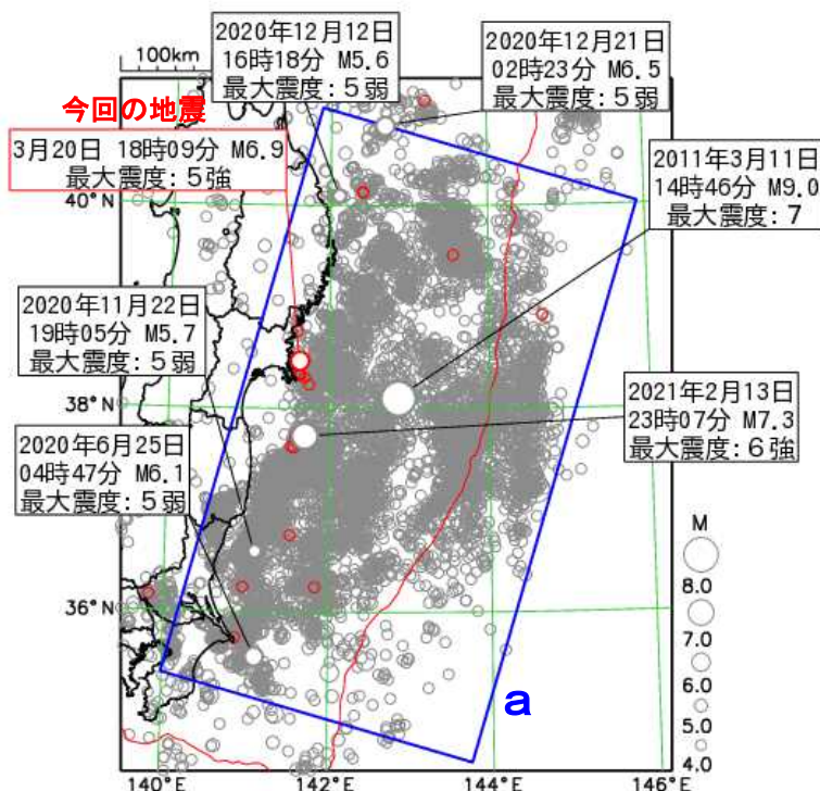
図2 震央分布図 (2011年3月1日～2021年3月31日 深さすべて M \geq 4.0) ※2021年3月の地震を赤で表示
