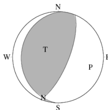
図3 下半球等積投影 CMT解 3月20日18時09分 (M6.9)
