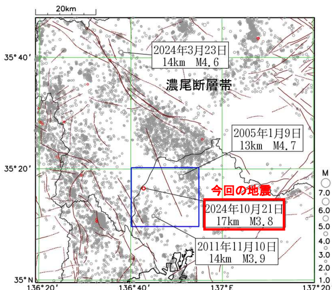
図 2 震央分布図
