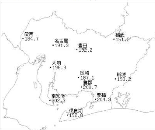
アメダス月別値 2023年12月 日照時間(h)
