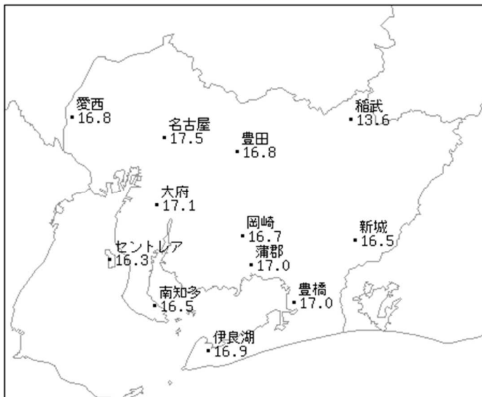
アメダス月別値 2024年4月 平均気温(°C)
