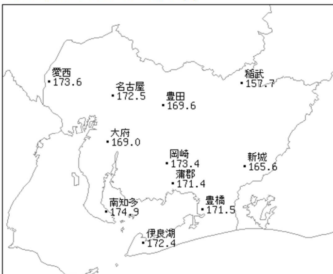
アメダス月別値 2024年4月 日照時間(h)
