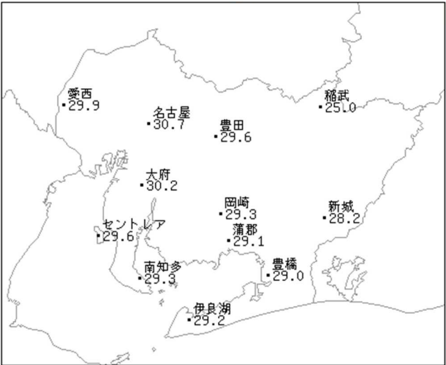
アメダス月別値 2025年8月 平均気温(°C)
