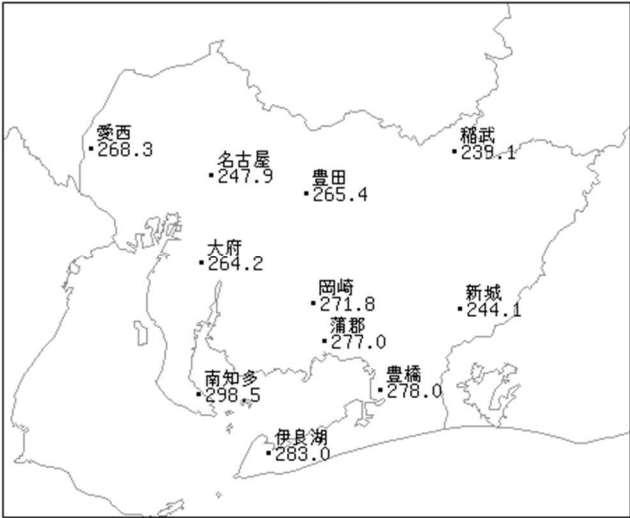
アメダス月別値 2025年8月 日照時間(h)
