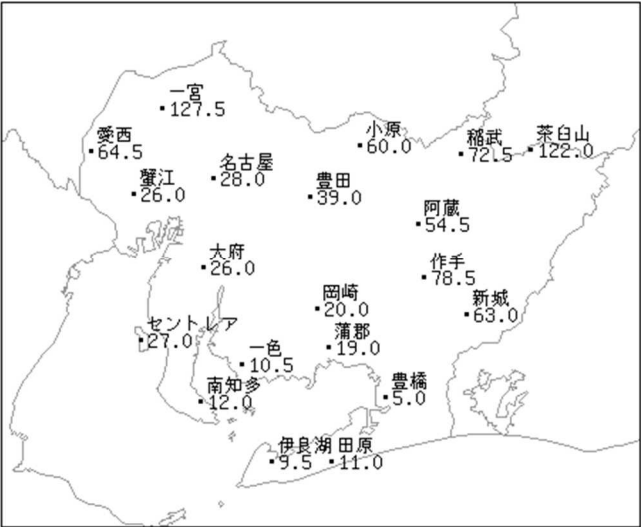
アメダス月別値 2025年8月 降水量(mm)
