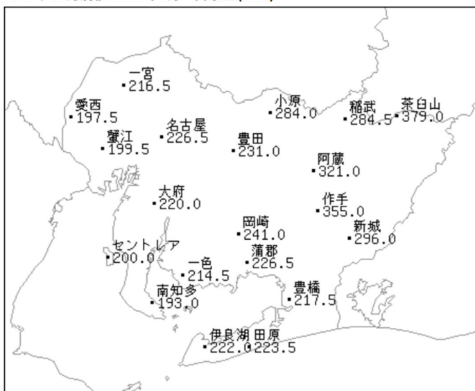
アメダス月別値 2026年4月 日照時間(h)
