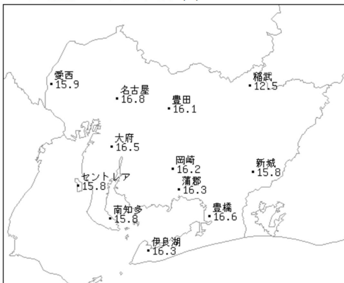
アメダス月別値 2026年4月 平均気温(°C)
