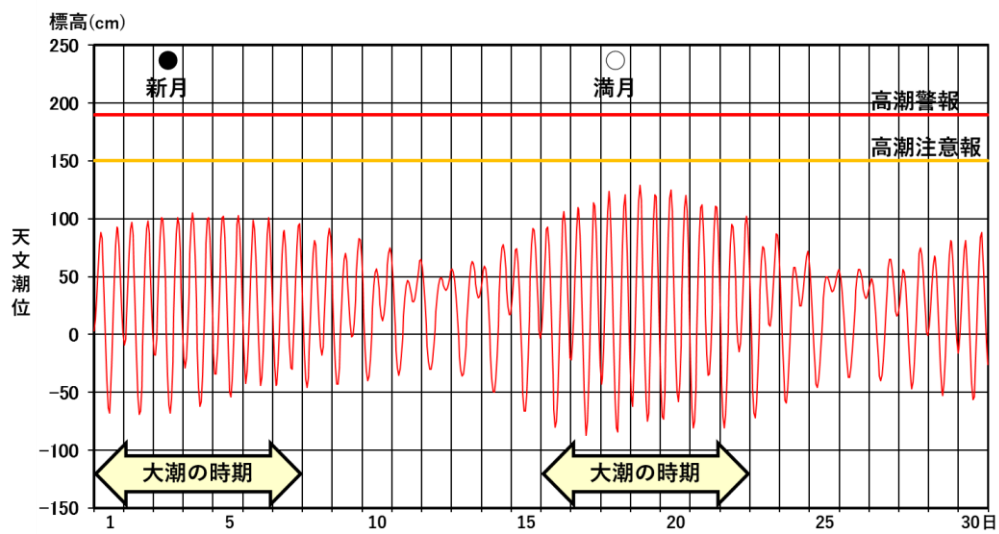
図3 奄美における2024年9月（1時間ごとの）の天文潮位
