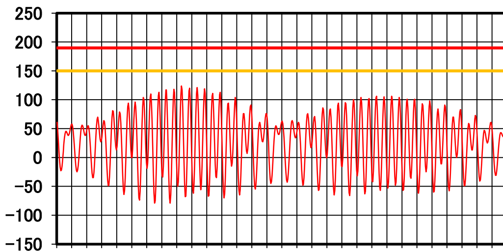
図3 奄美における 2025 年 9 月(1時間ごとの)の天文潮位
