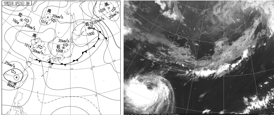
8月25日03時の地上天気図（左）と気象衛星赤外面像（右）
