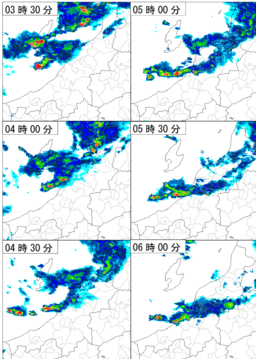
1 2 4 8 12 16 24 32 40 48 56 64 80 < mm/h 8月25日03時30分から30分毎のレーダー画像
