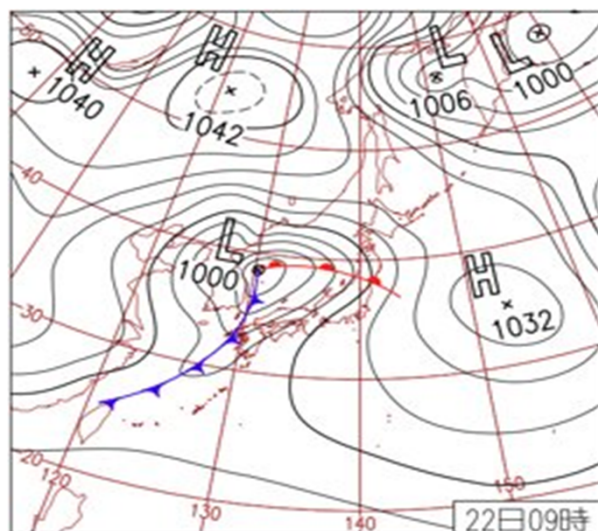
地上天気図 平成28年12月22日9時
