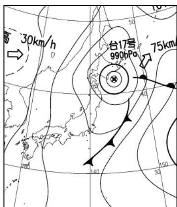
地上天気図
