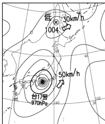
地上天気図
