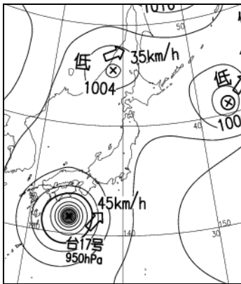
地上天気図
