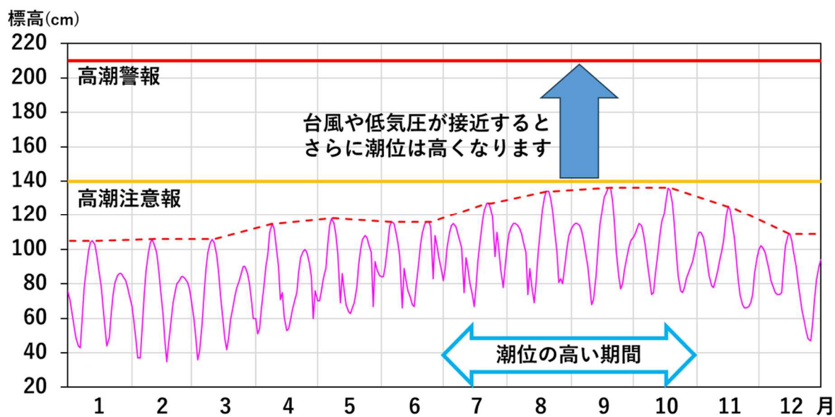
図2 大分における2024年の天文潮位の日最高値
