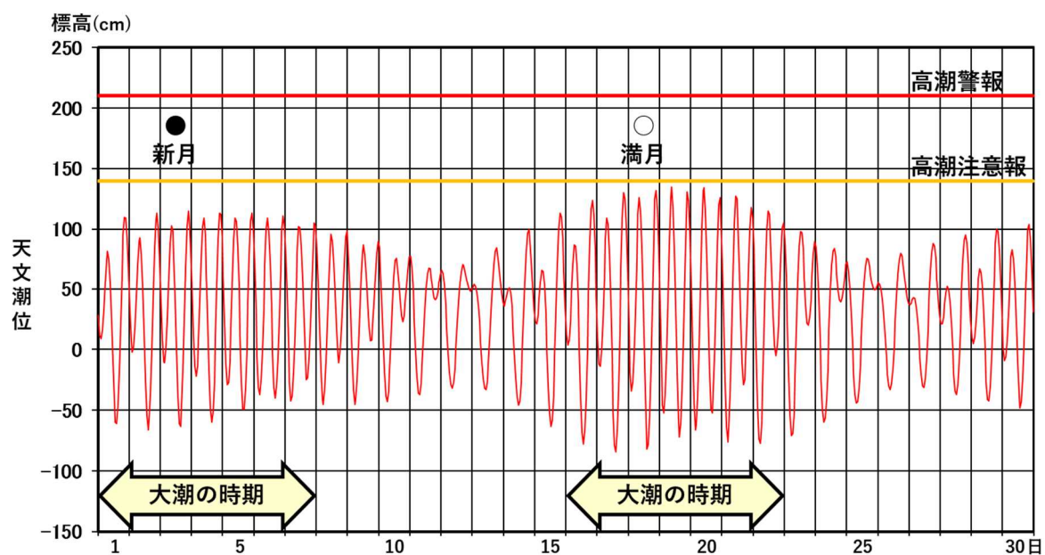
図3 大分における2024年9月（1時間ごとの）の天文潮位
