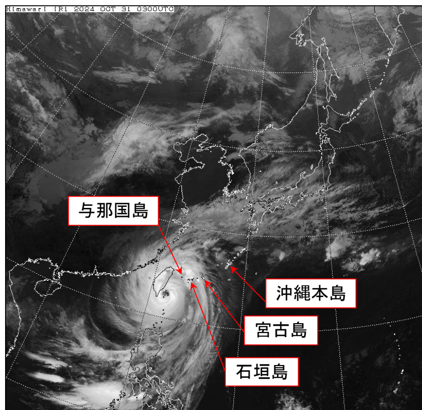
気象衛星画像（赤外） 2024年10月31日12時
