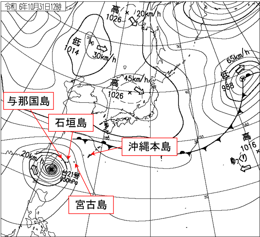
地上天気図 2024年10月31日12時
