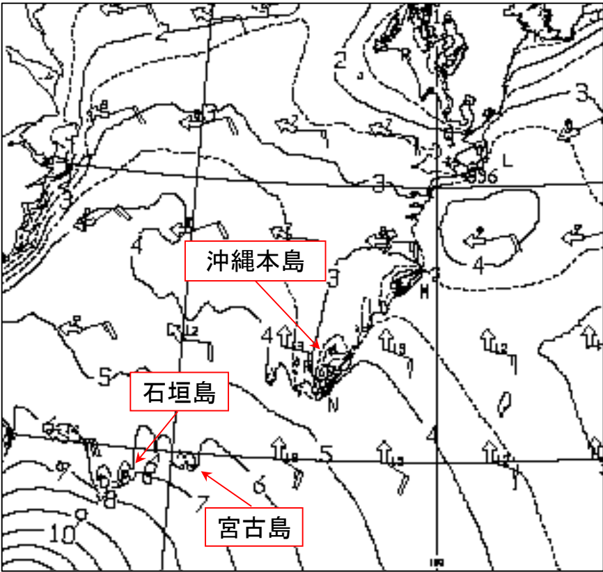
沿岸波浪実況図 2024年10月31日9時
