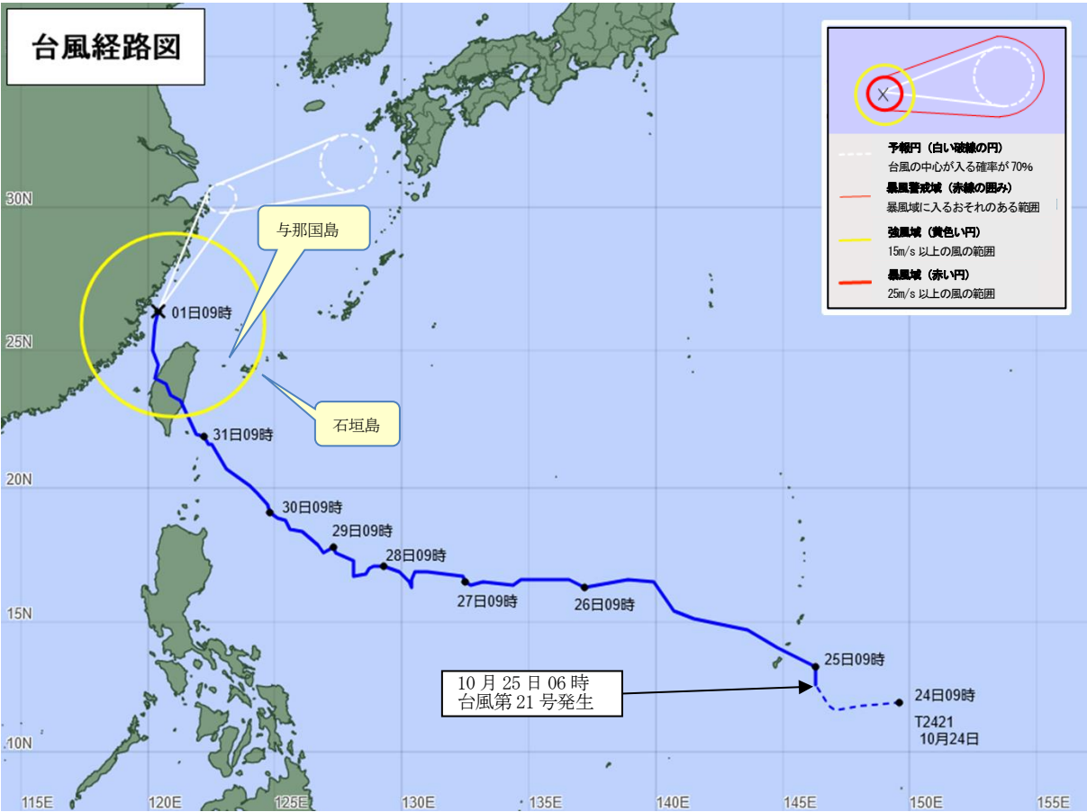
台風第21号経路図（2024年11月1日09時現在 速報値）
