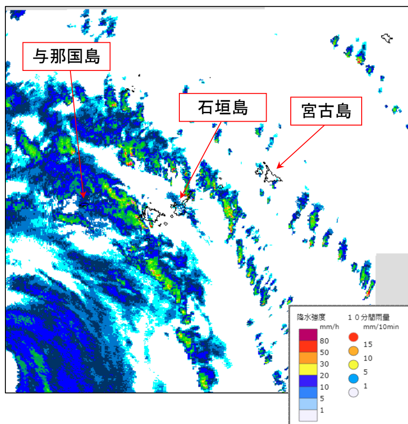
気象レーダー画像（降水強度） 2024年10月31日12時
