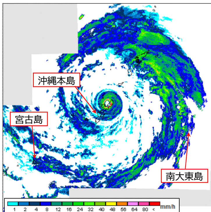
気象レーダー画像（降水強度） 2026年8月7日15時
