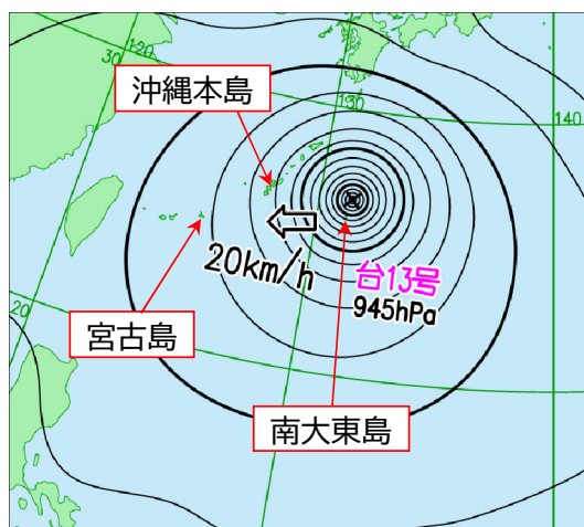
地上天気図 2026年8月6日21時
