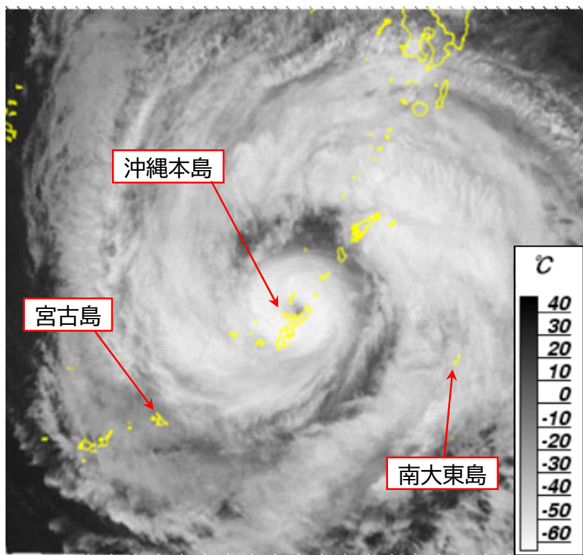
気象衛星画像（赤外） 2026年8月7日15時
