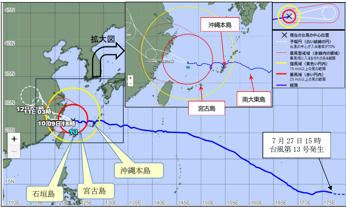
台風第13号経路図（2026年8月9日6時現在 速報）
