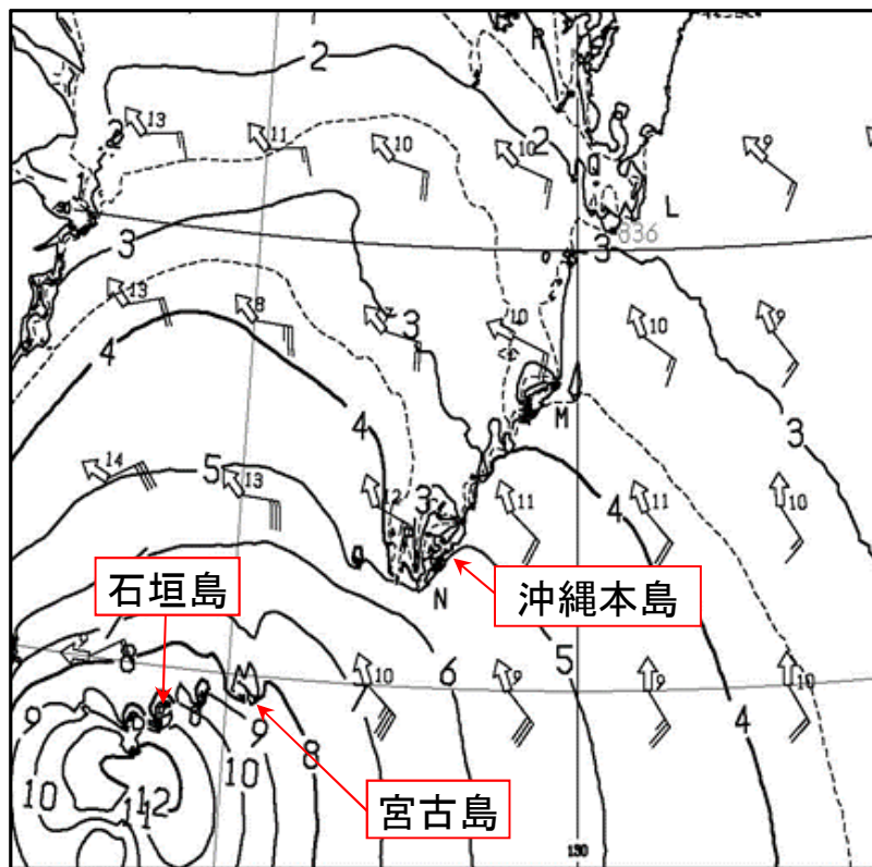
沿岸波浪実況図 2016年9月27日09時
