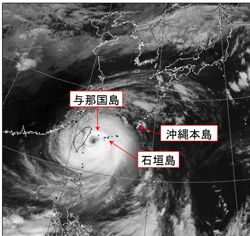
気象衛星画像（赤外）2016年9月27日12時
