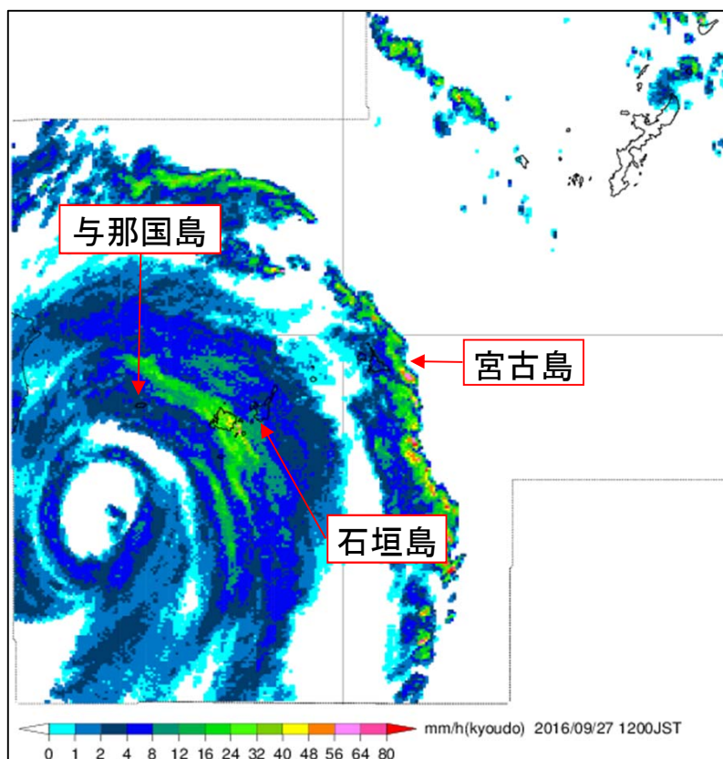
気象レーダー（降水強度）2016年9月27日12時
