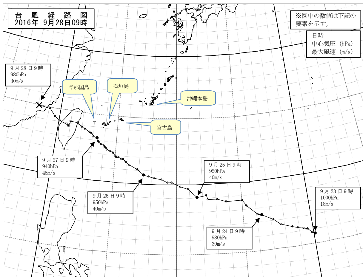
台風第17号経路図（2016年9月28日09時現在 速報値）
