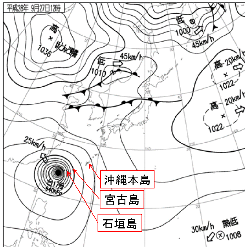
地上天気図 2016年9月27日12時
