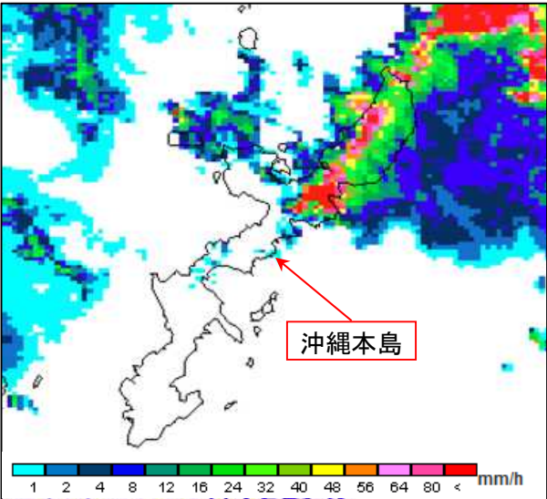
降水強度11月9日01時30分
