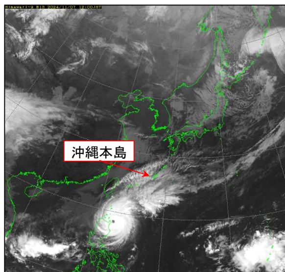
気象衛星画像(赤外) 11月7日9時
