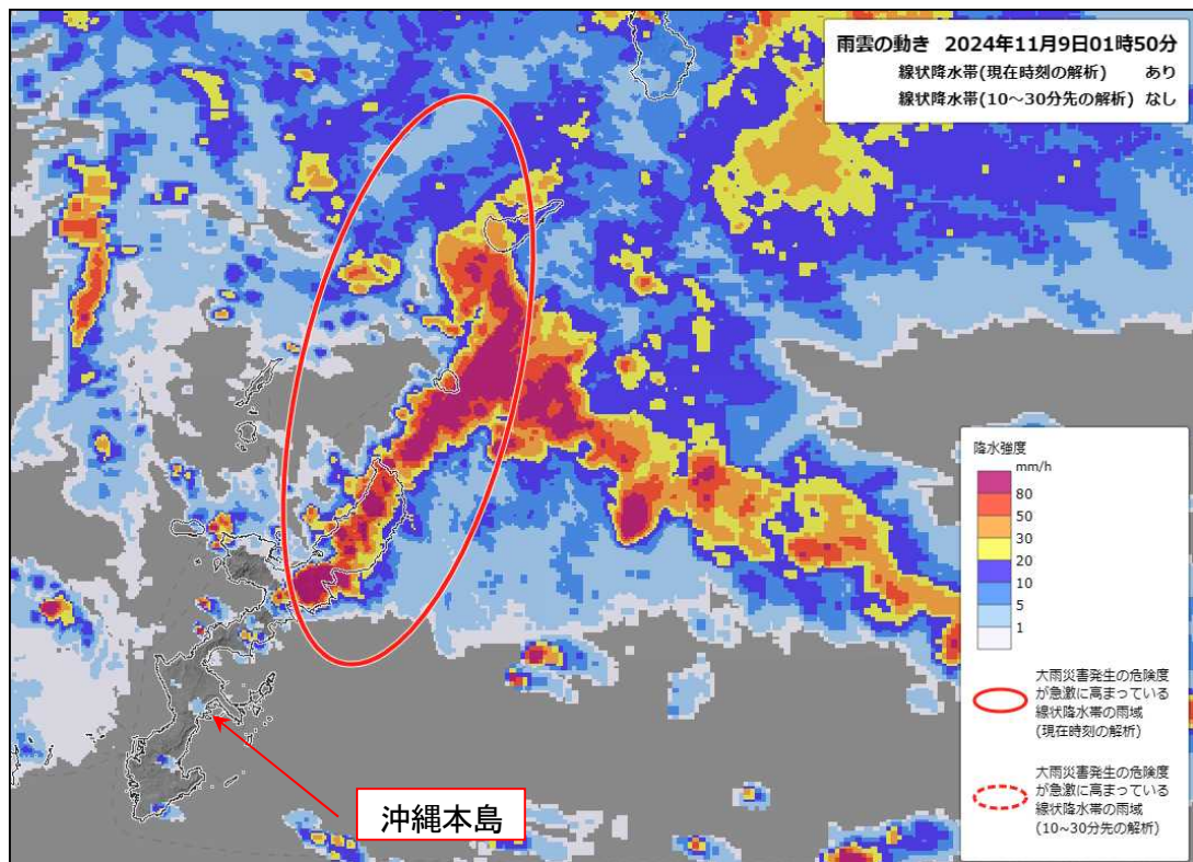
図1 降水ナウキャスト（雨雲の動き・線状降水帯（現在時刻の解析）11月9日01時50分）
