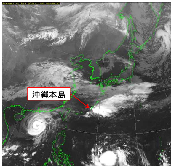
気象衛星画像(赤外) 11月9日9時
