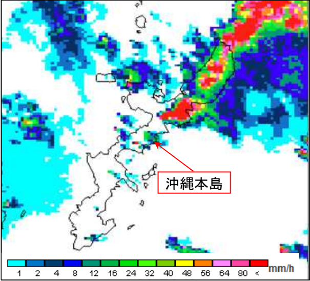
降水強度 11月9日02時00分
