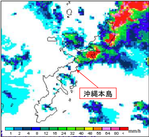
降水強度 11月9日02時30分
