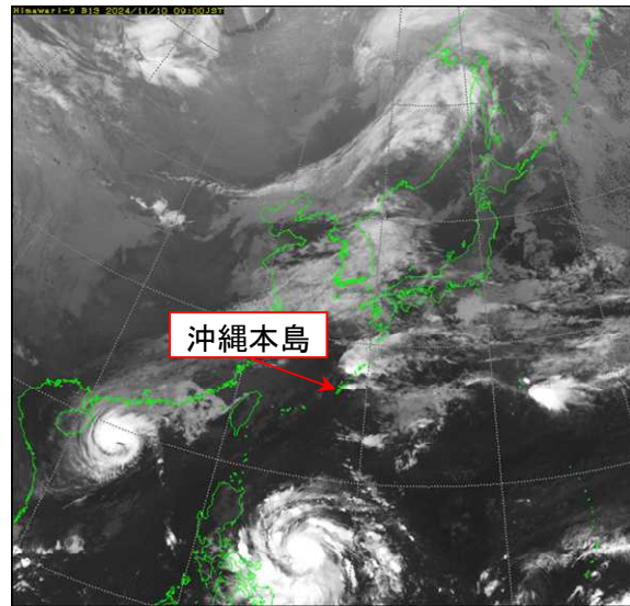
気象衛星画像(赤外) 11月10日9時
