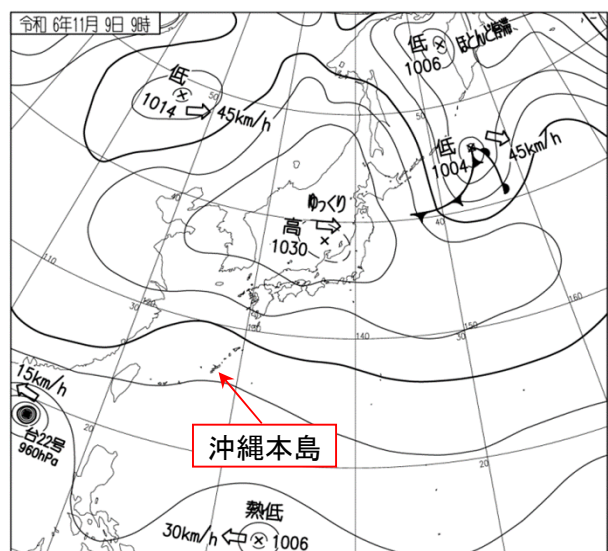
地上天気図 11月9日9時
