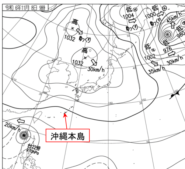
地上天気図 11月8日9時
