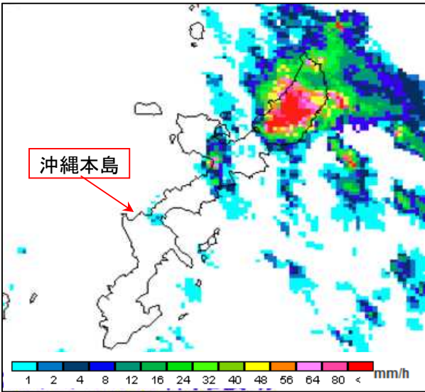
降水強度 11月10日05時30分
