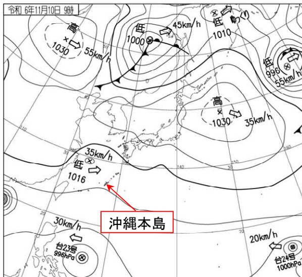
地上天気図 11月10日9時
