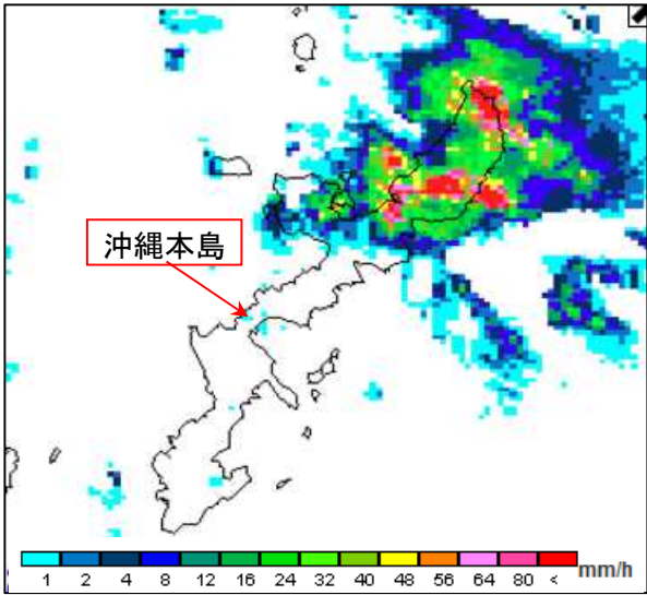
降水強度 11月10日06時30分
