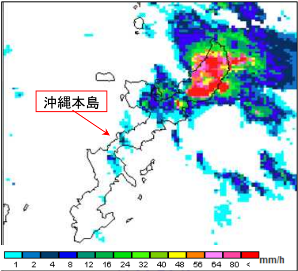
降水強度 11月10日06時00分
