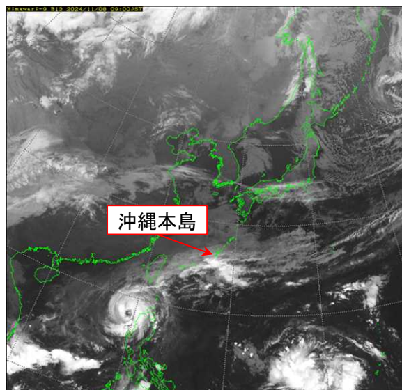
気象衛星画像(赤外) 11月8日9時
