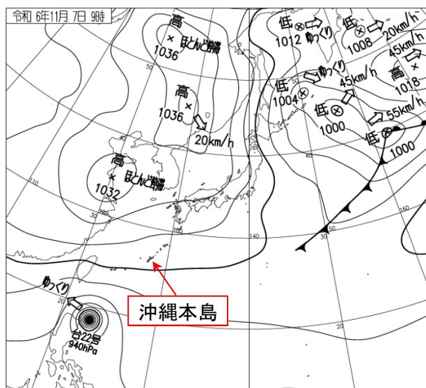
地上天気図 11月7日9時
