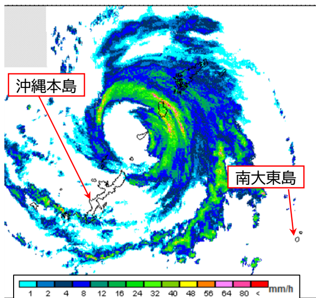
気象レーダー降水強度 2026年8月26日0時
