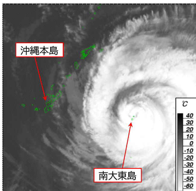
気象衛星画像（赤外） 2026年8月25日8時
