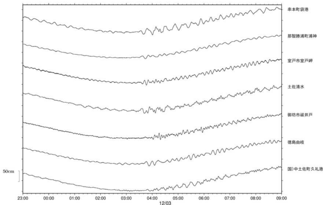
津波波形図
